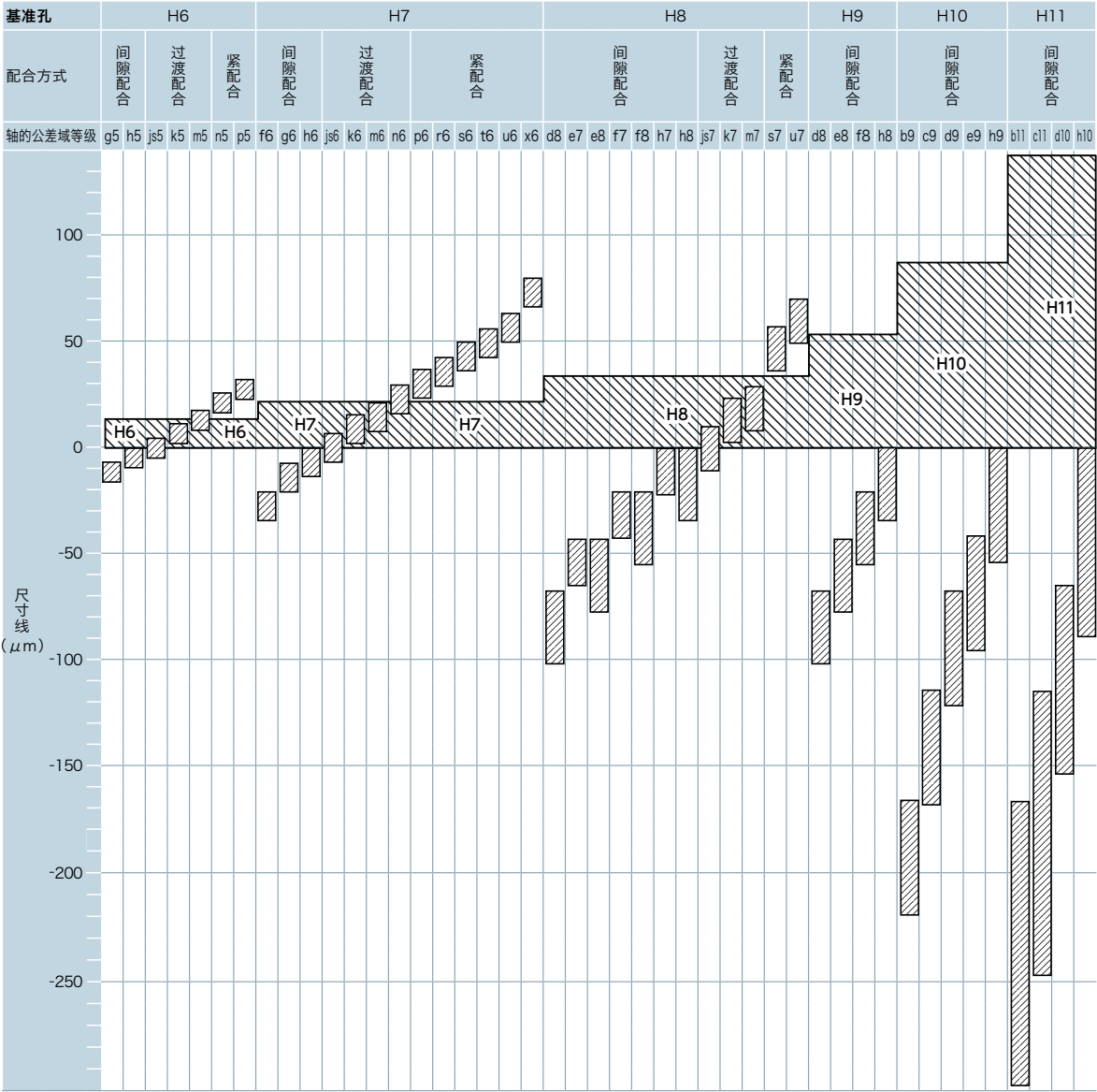
常用的孔基准配合时公差域分类的相互关系
