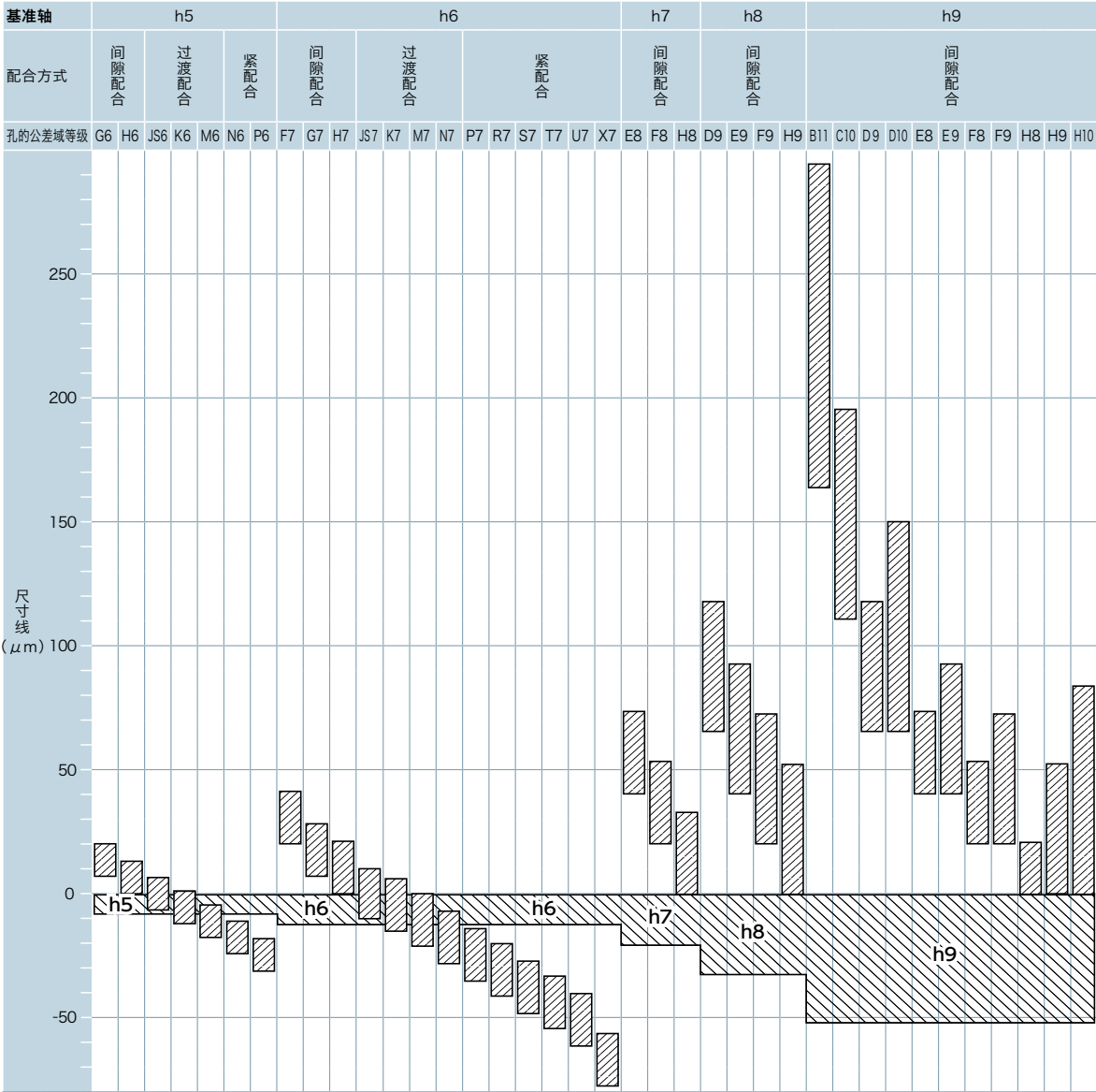
常用的轴基准配合时公差域分类的相互关系
