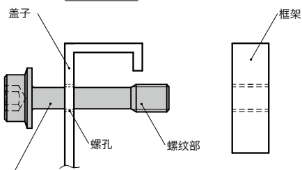
SSC-SFSS 带法兰内六角防脱落螺丝
