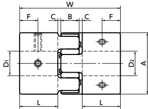
外径 φ55-φ95
