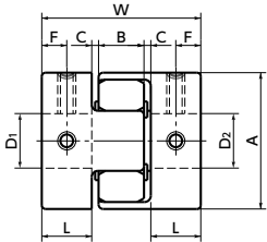
外径 φ14-φ30
