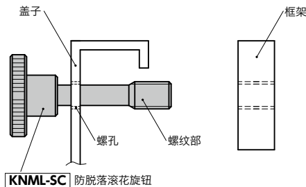
KNML-SC 防脱落滚花旋钮
