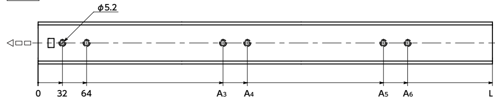
外滑轨
