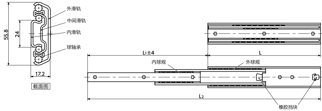
外滑轨
